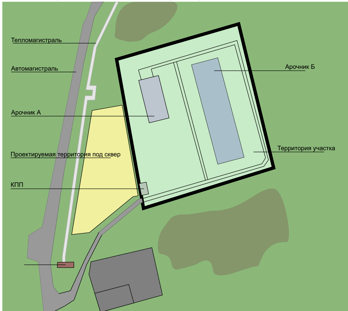
План схема расположения объектов проектирования
